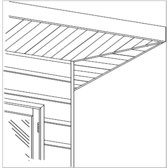
Fig 20a Soffit Detail
