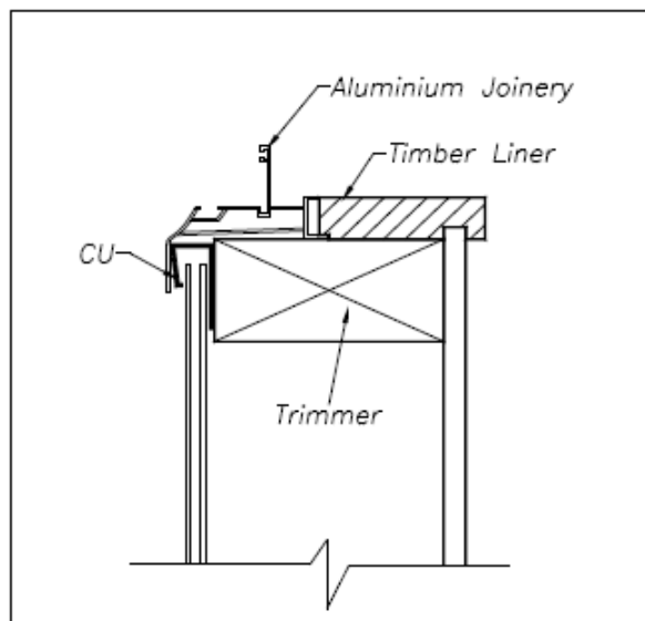
Fig 8 Jamb
